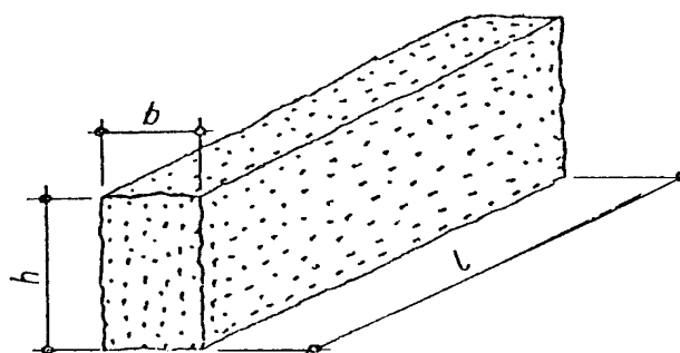
Rys. 6. Krawężnik drogowy Tablica 4. Wymiary
